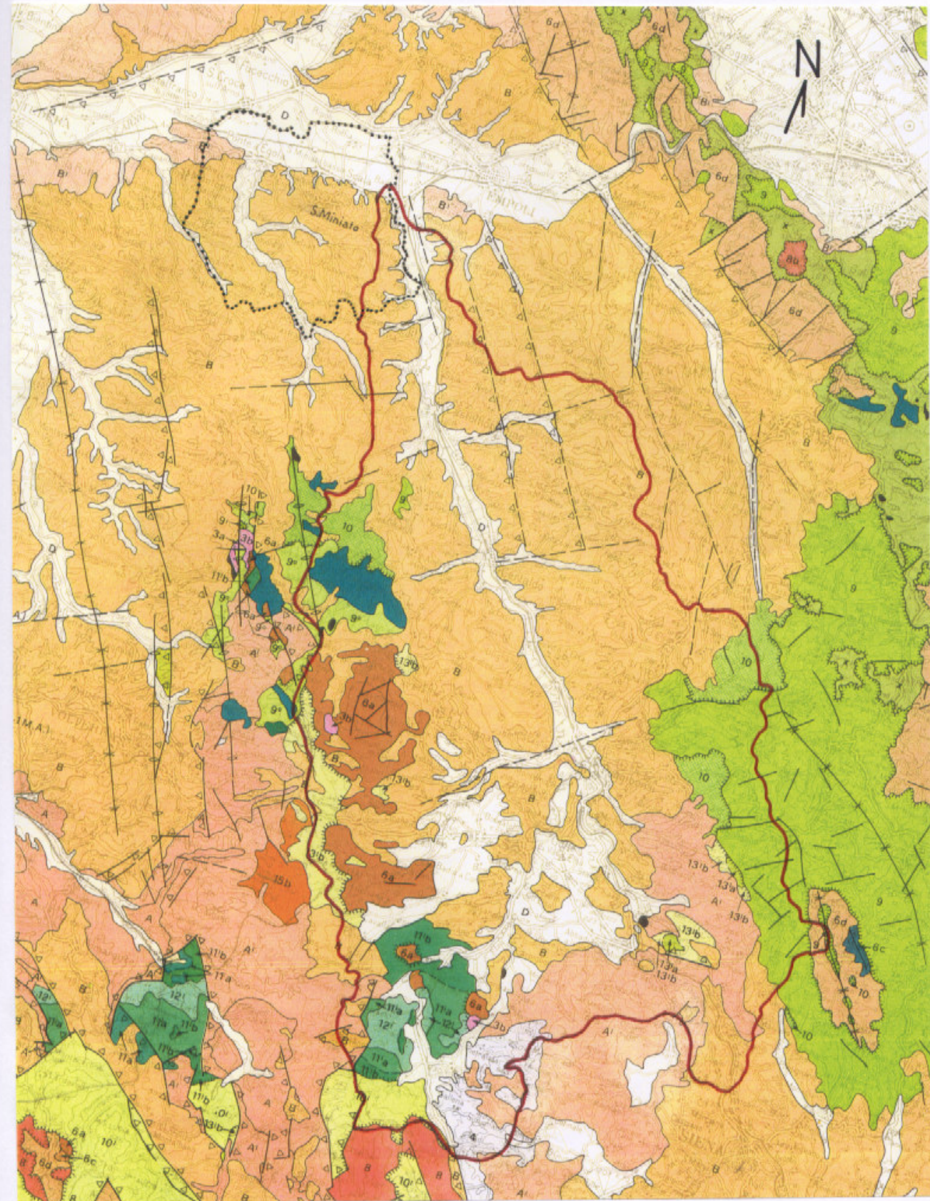
ALLEGATO N.1: schema strutturale - scala 1:250.000 (Progetto Finalizzato Geodinamica - CNR. Abbate E. et Alii 1982)
